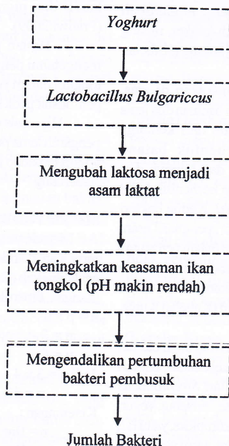
Gambar 1. Kerangka konsep
