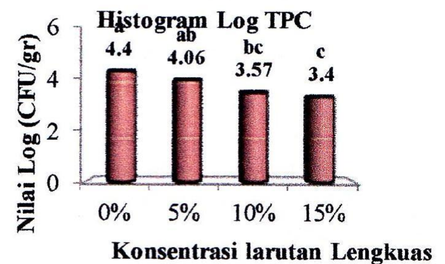
Gambar 2 Histogram nilai TPC ikan kembung.
