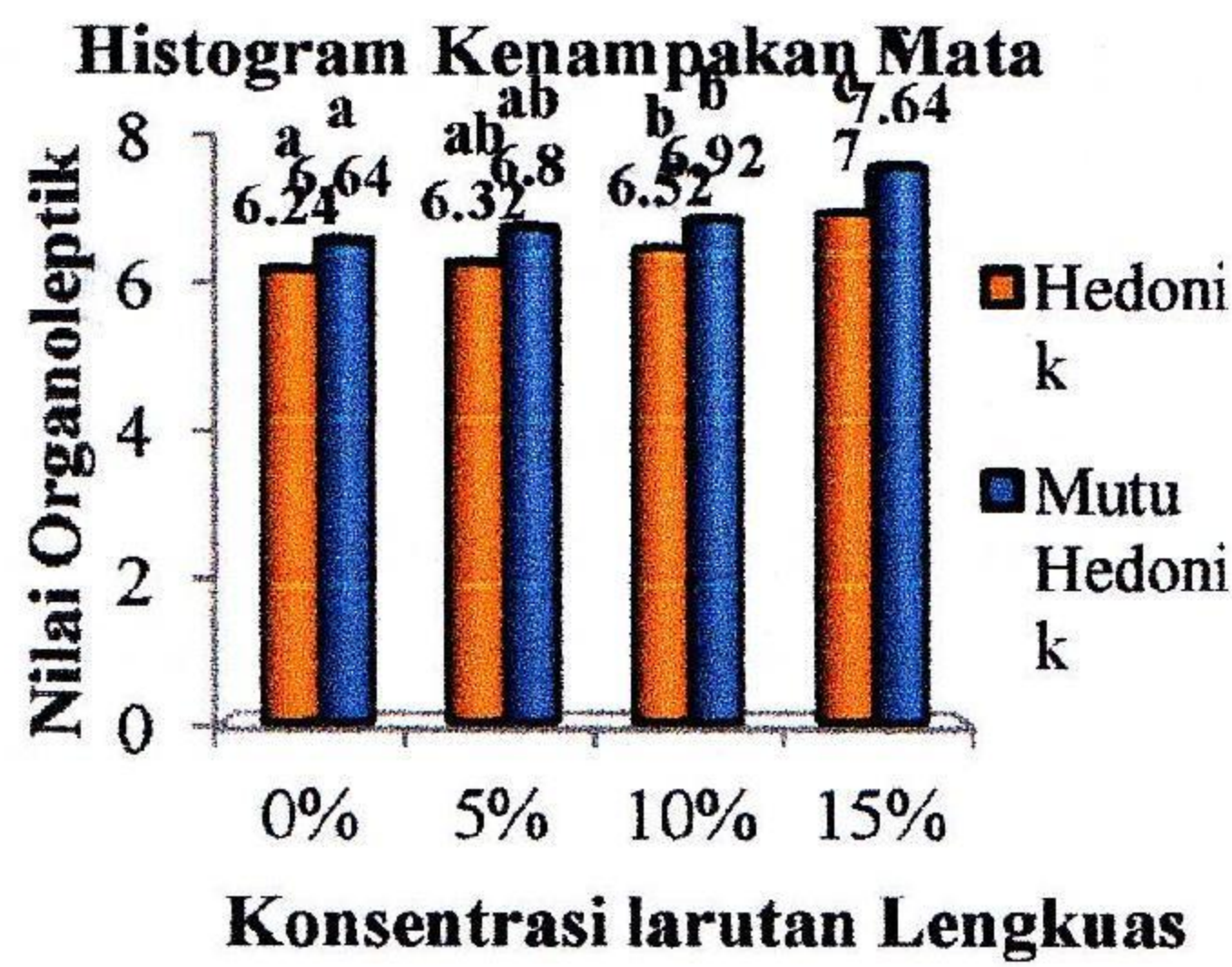
Gambar 1 Histogram nilai organoleptik mata ikan kembung.
