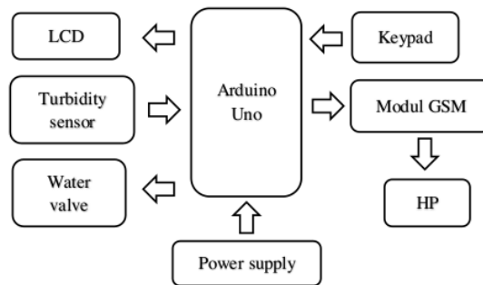
Gambar 1. Blok Diagram Sistem Katup Cerdas
