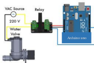
Gambar 5. Koneksi Water Valve dengan Arduino
