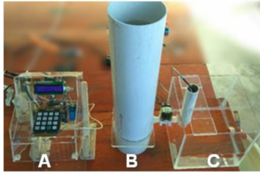
Gambar 9. Model katup cerdas
