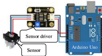
Gambar 3. Koneksi Turbidity Sensor dan Arduino
