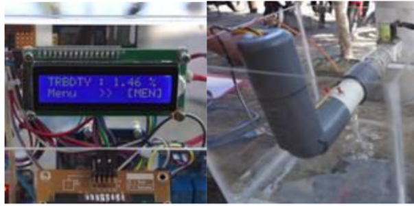
Gambar 11. Hasil Pengujian dengan Air Bersih atau Jernih
