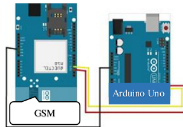
Gambar 4. Koneksi Modul GSM dan Arduino
