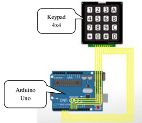
Gambar 6. Koneksi Arduino Uno dengan keypad 4x4
