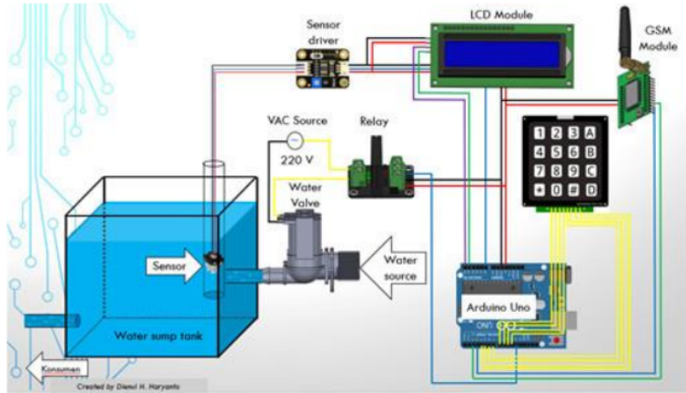
Gambar 2. Skema Perancangan Perangkat Keras
