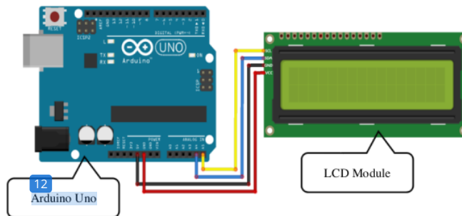
Gambar 7. Koneksi Arduino Uno dan LCD Module
