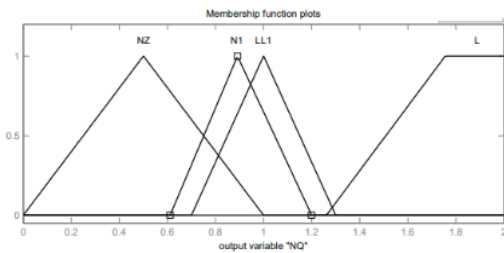
Gambar 8. Grafik Fungsi keanggotaan keluaran q
