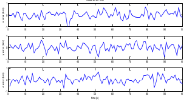
Gambar 4. Grafik galat lintasan target hasil pengukuran
