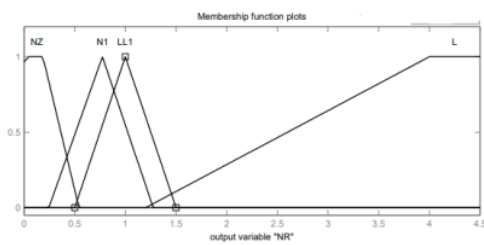
Gambar 9. Grafik fungsi keanggotaan keluaran r
