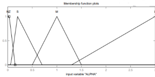
Gambar 7. Grafik fungsi keanggotaan masukan
