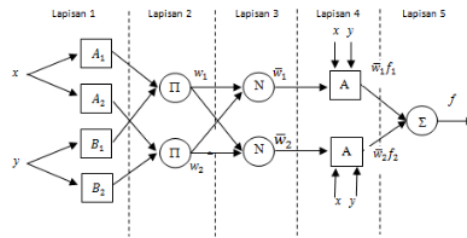
Gambar 2. Arsitektur jaringan ANFIS
