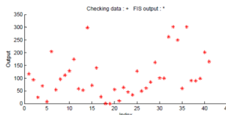
Gambar 8. Hasil testing model ANFIS untuk data membukit
