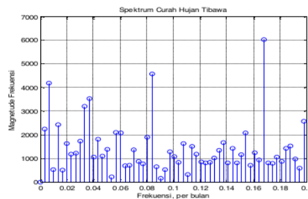
Gambar 5. Spektrum Frekuensi tanpa Frekuensi Nol
