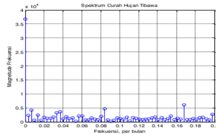
Gambar 4. Spektrum Frekuensi Data Curah Hujan Tibawa
