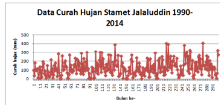
Gambar 3. Data Curah Hujan Stamet Jalaluddin
