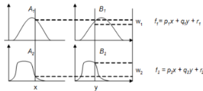
Gambar 1. ANFIS Sugeno orde satu
