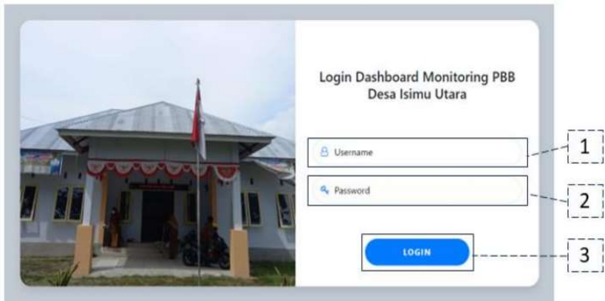
Gambar 4 halaman login
