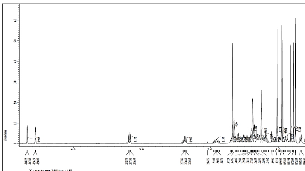
Gambar 3. Spektrum H-NMR isolat murni
