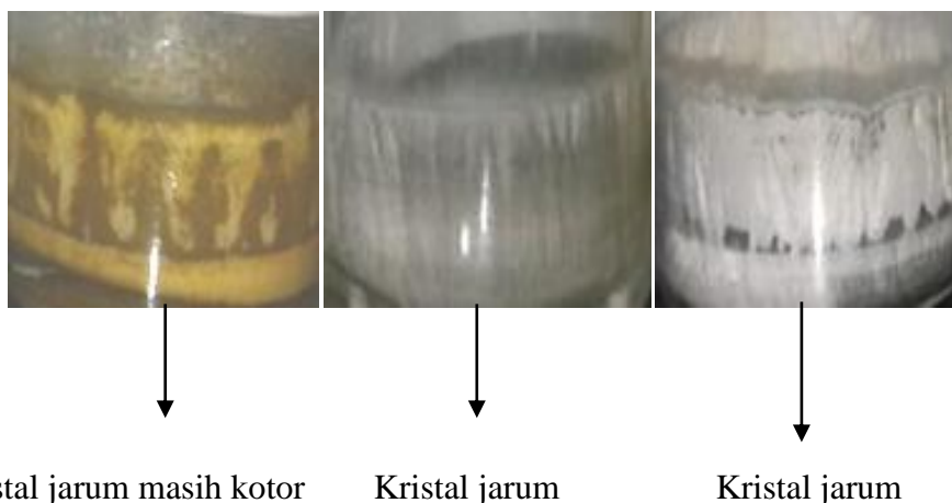
Gambar 1. Profil fraksi C yang ada kristal jarum berwarna putih
