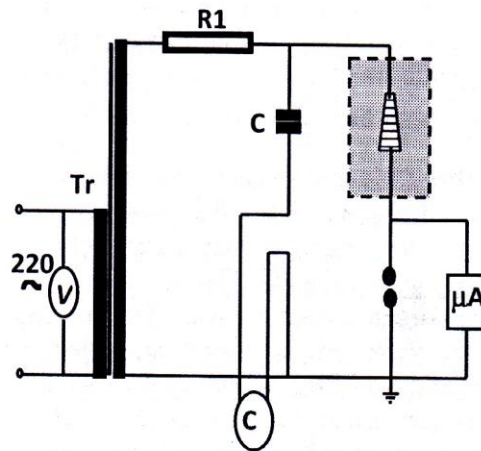
Gambar 1. Skema pengukuran arus bocor pada isolator uji
