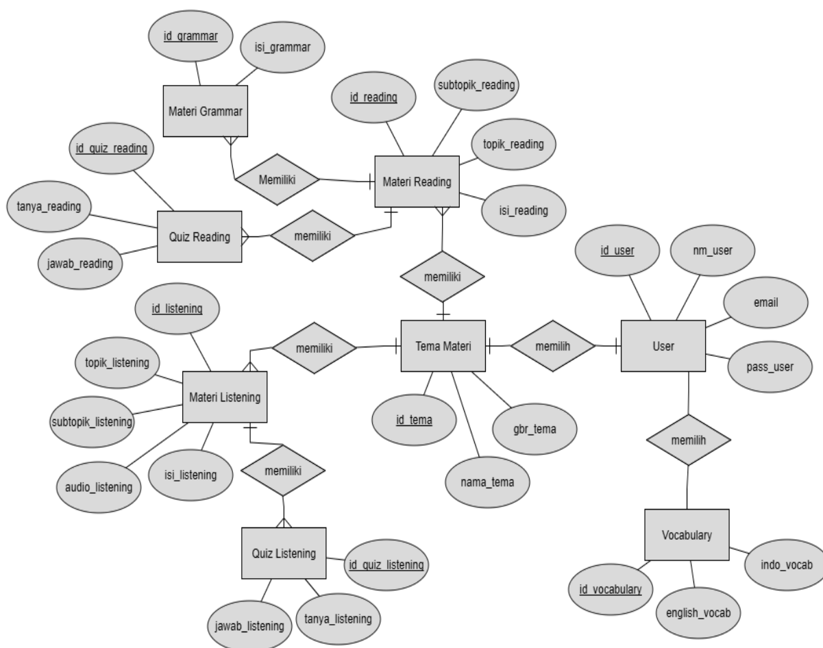
Gbr. 3 ERD aplikasi MALL yang dikembangkan.
