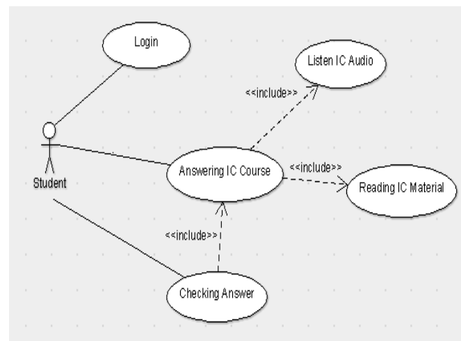
Gbr. 1 Diagram use case pada aplikasi WBCALL yang telah dikembangkan sebelumnya [12].
