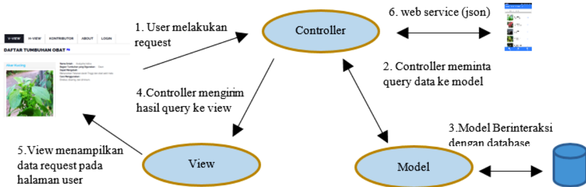
Gambar 4. Arsitektur aplikasi
