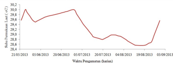
Variasi suhu permukaan laut (SPL) di sekitar Manokwari pada Bulan Mei sampai Agustus 2013.
