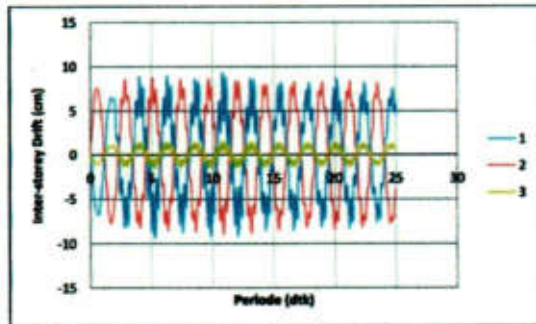
Gambar 9. Nilai inter-storey drift ketika mesin berada pada lantai pertama
