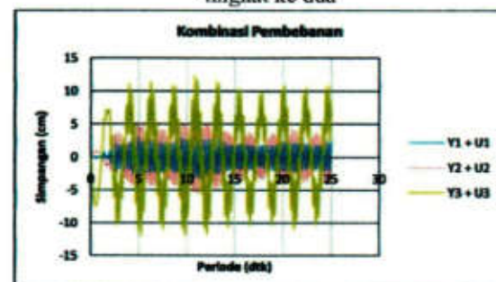
Gambar 7. Respon struktur akibat getaran mesin pada tingkat ke dua
