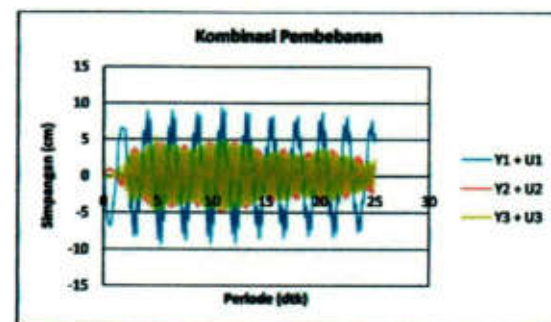
Gambar 6. Respon struktur akibat getaran mesin pada tingkat pertama
