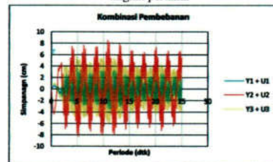
Gambar 7. Respon struktur akibat getaran mesin pada tingkat ke dua
