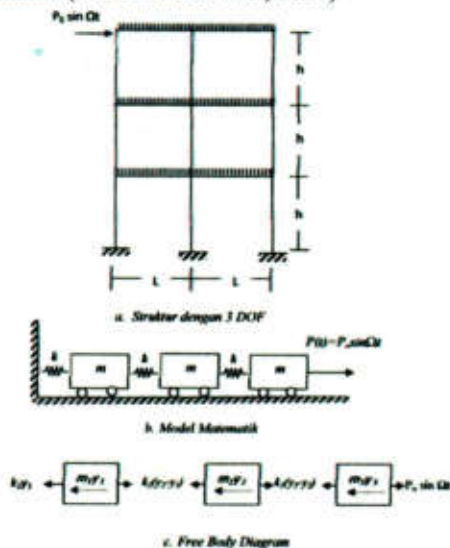
Gambar 5. Struktur dengan Pembebanan Harmonis
