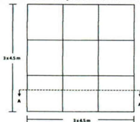
Gambar 1. Denah Struktur Portal
