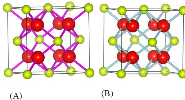
Gambar 1 Struktur CeO 2 ; (A) sebelum simulasi jarak Ce-O = 2,34313 Å dan (B) setelah disimulasi menggunakan GULP dengan jarak Ce-O = 2,34257 Å
