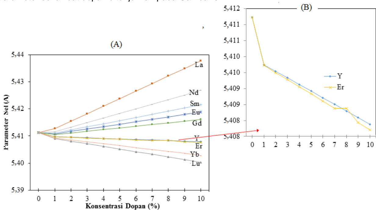
Gambar 3 Parameter CeO 2 yang didoping dengan kation trivalen
