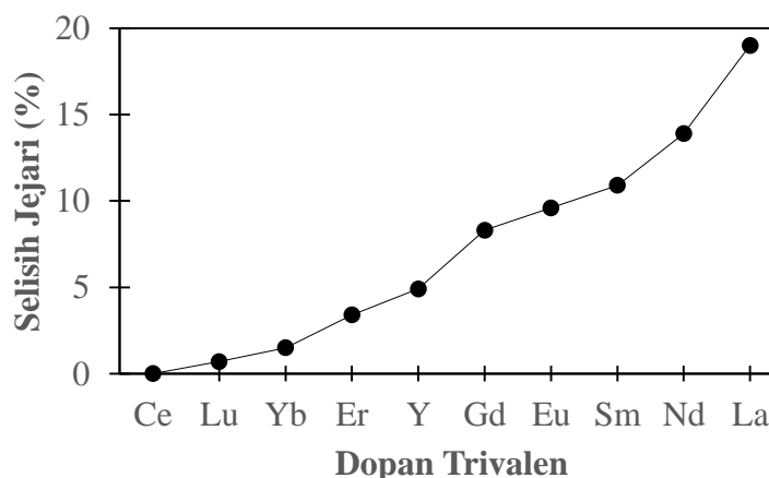
Gambar 2. Selisih jari-jari dopan trivalen terhadap kation host Ce 4+
