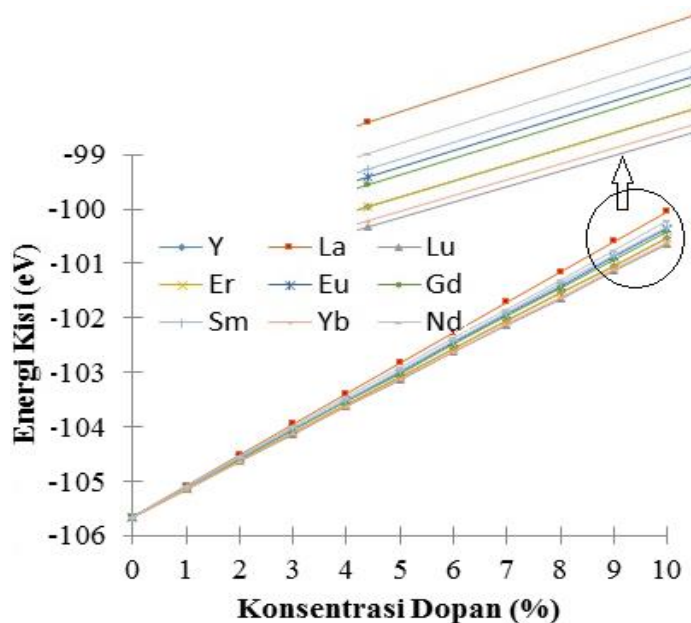
Gambar 4 Energi kisi CeO 2 yang terdoping kation trivalen
