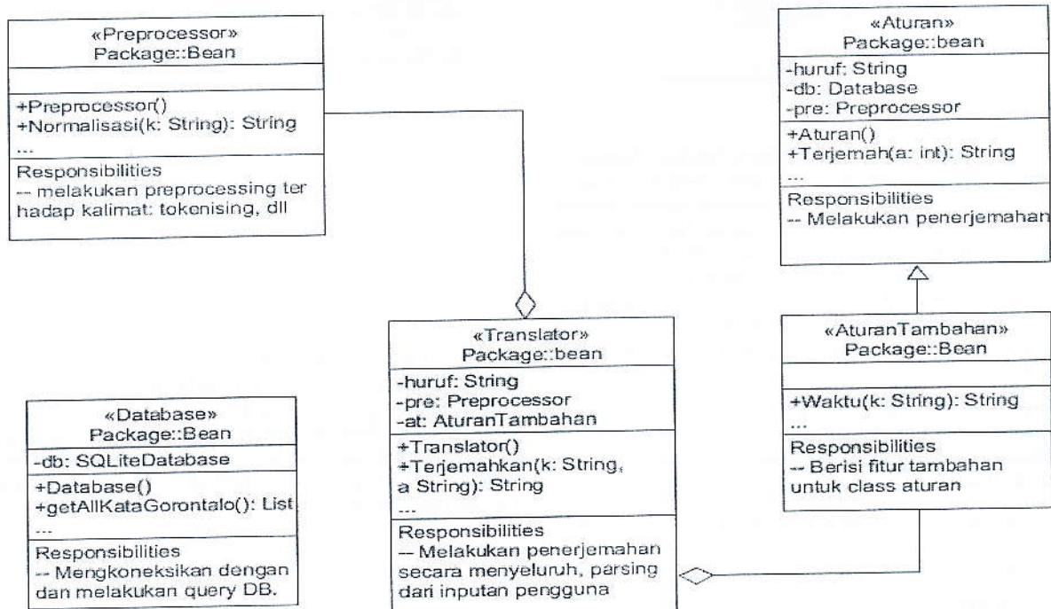
Gambar 1. Diagram kelas sistem penerjemahan
