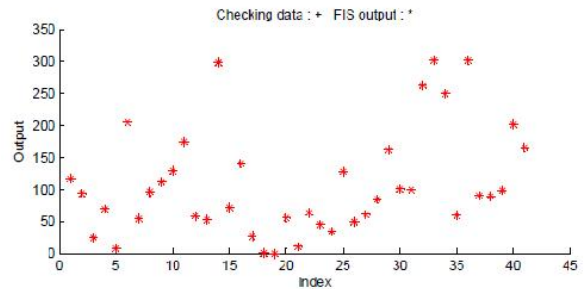
Gambar 10. Hasil testing model ANFIS untuk data membukit
