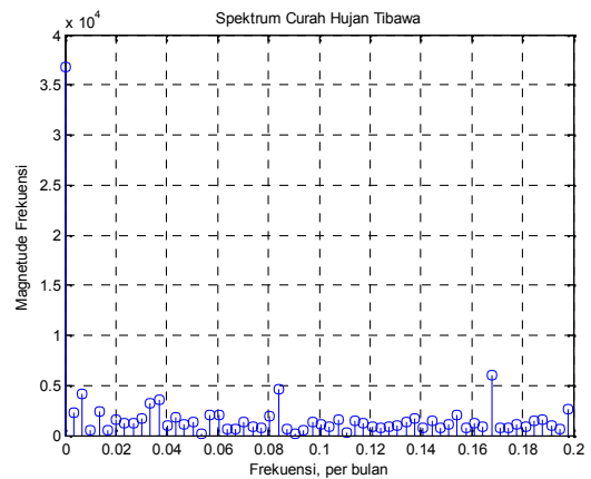
Gambar 3. Spektrum Frekuensi Data Curah Hujan Tibawa
