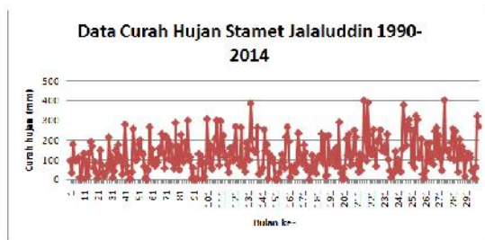
Gambar 2. Data Curah Hujan Stamet Jalaluddin
