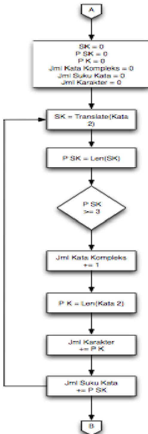
Gambar 2 : Lanjutan Flowchart Program
