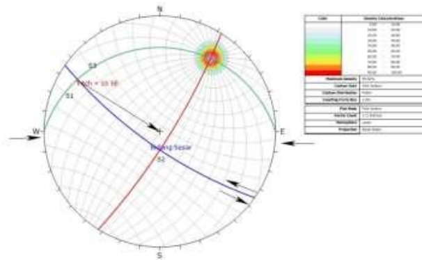
Gambar 6 pengolahan data struktur geologi
