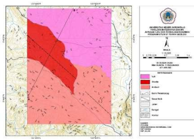
Gambar 7 Peta geologi Desa Labanu
