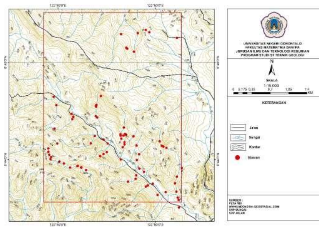
Gambar 2 peta kerangka geologi Desa Labanu Kec. Tibawa
