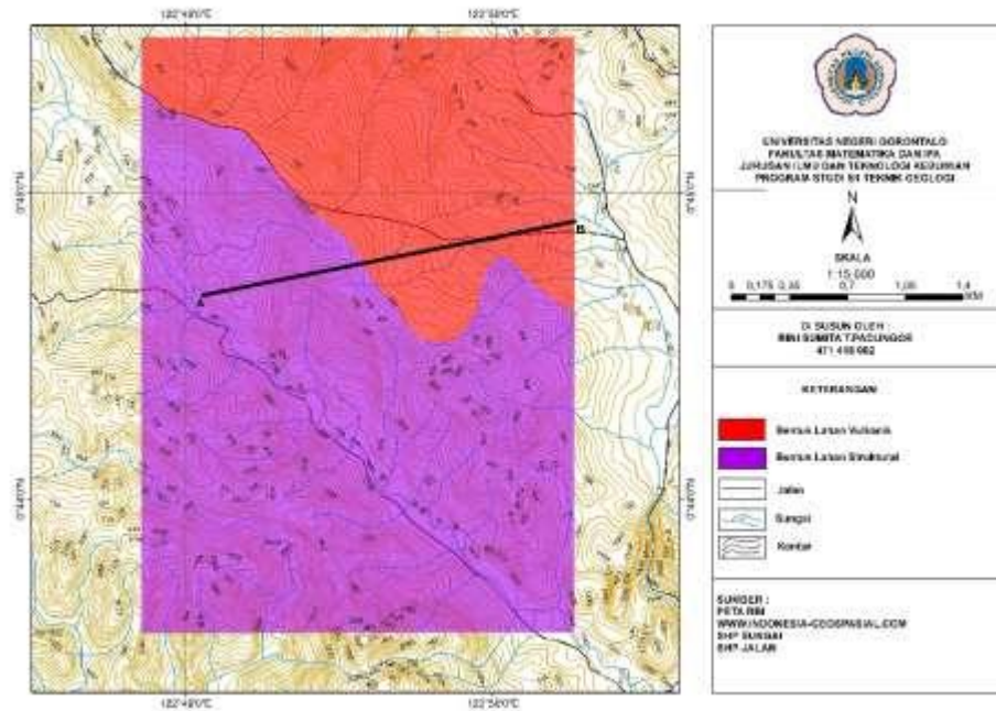
Gambar 3 Peta geomorfologi Desa Labanu
