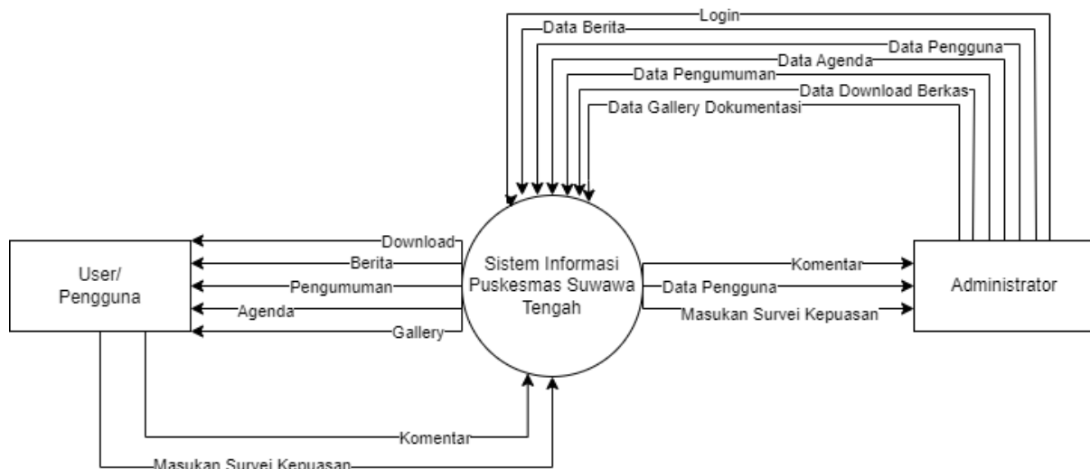
Gambar 4.1 Diagram Konteks
