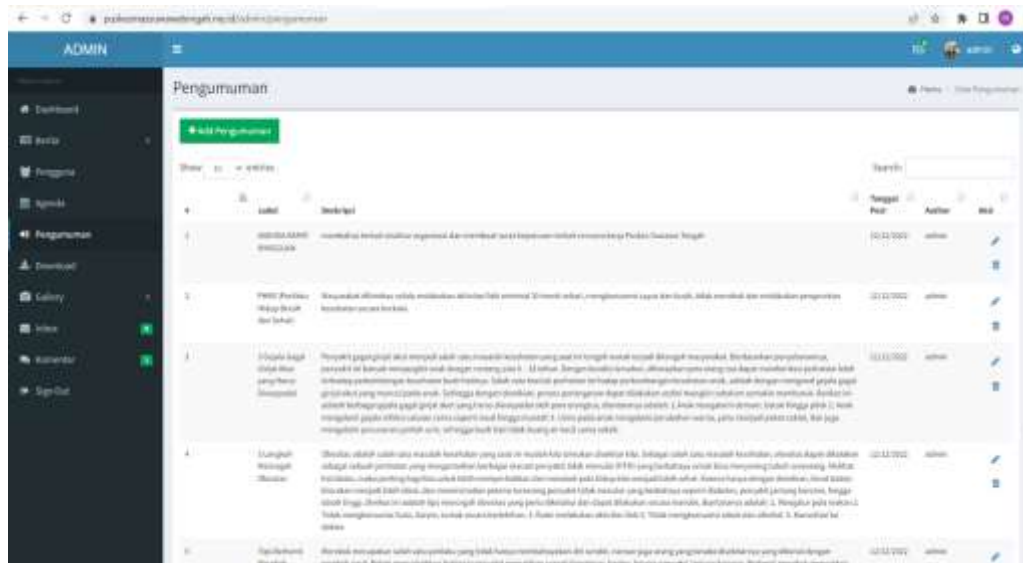
Gambar 4. 15 Tampilan Pengumuman
