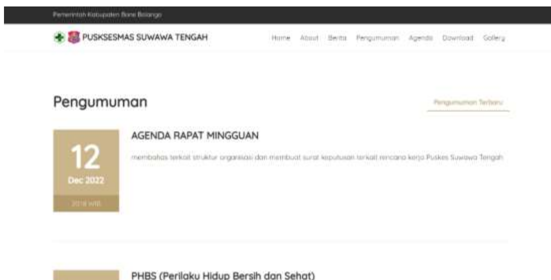
Gambar 4. 14 Tampilan Pengumuman
