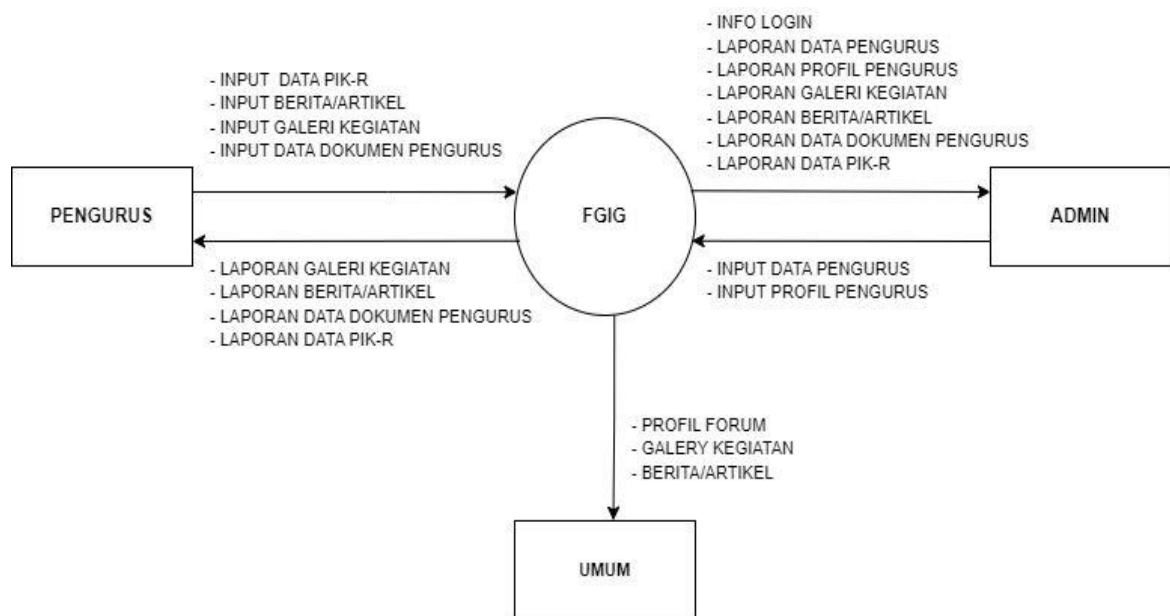
Gambar 1 . Diagram Konteks
